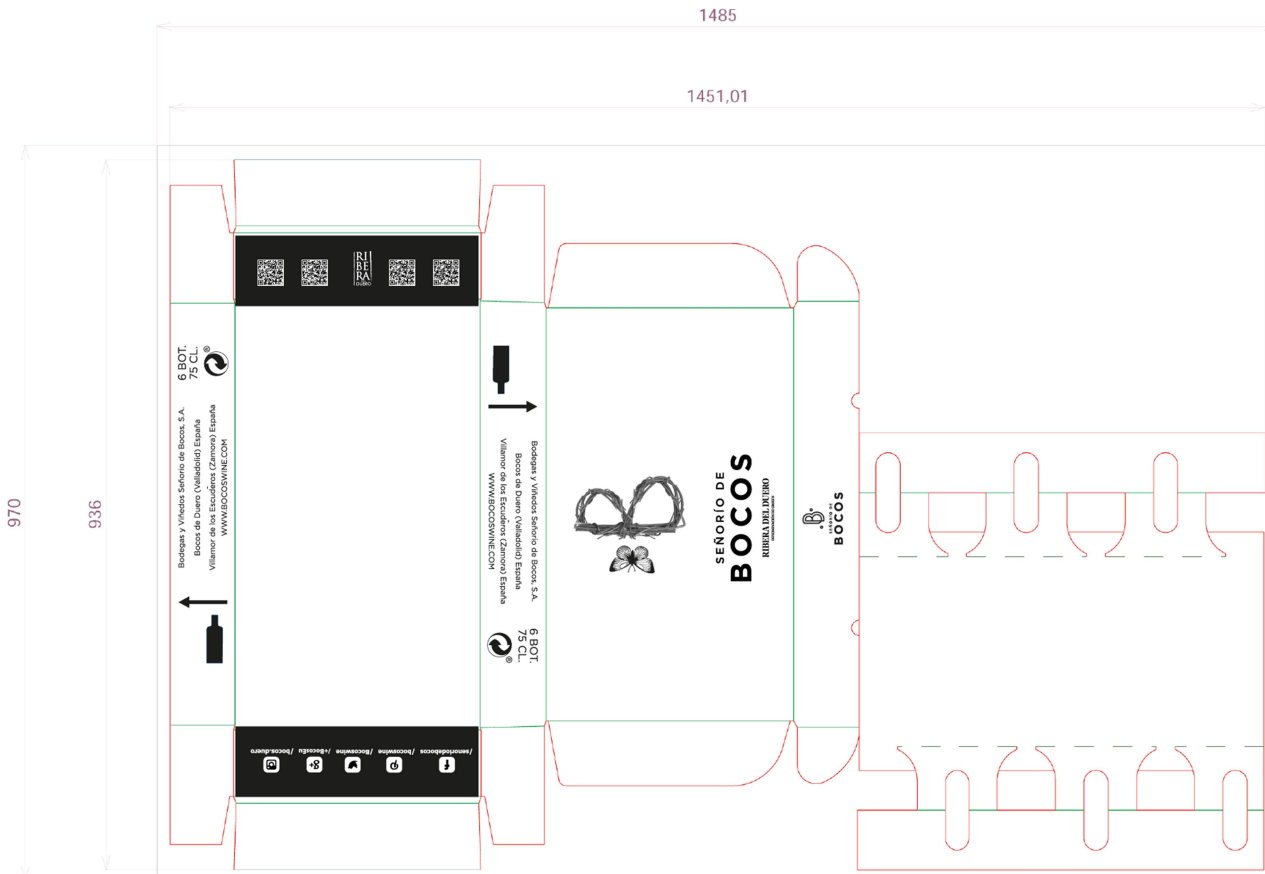
Troquel de la Caja de cartón contenedora de 6 botellas de 75 cl.
